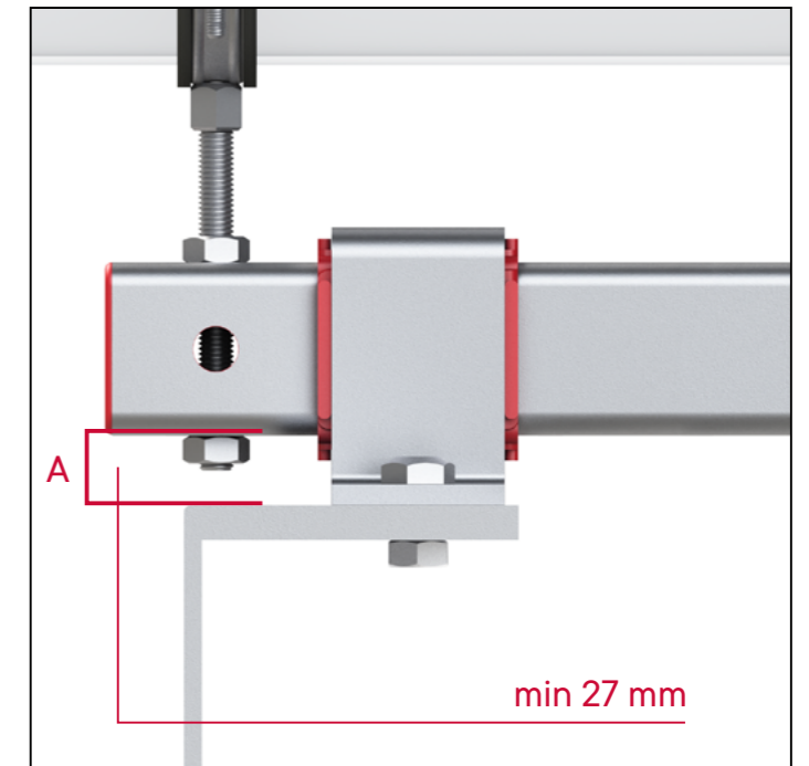
Увеличенная зона (A) для крепления шпильки. Нет ограничения перемещения подвижной части опоры при установки на широкое основание.
