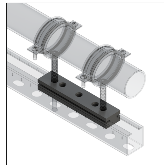
Большие перемещения, ограниченные только длиной профиля
