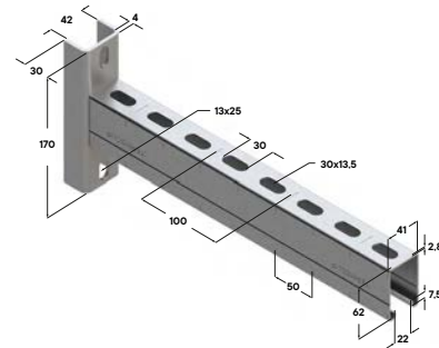
41x62 седельная
