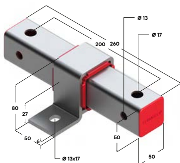
Опора скользящая TSA B50x50 F4
