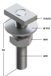
Болт Т-образный TBT 28 4F
