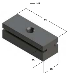
Опора скользящая TSE 28 F1
