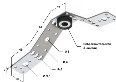
Кронштейн A-образный TDA 2F
