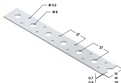
Металлическая перфорированная лента ЛС 1
