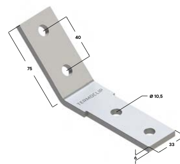
Уголок TA 45° 38-41 6F4
