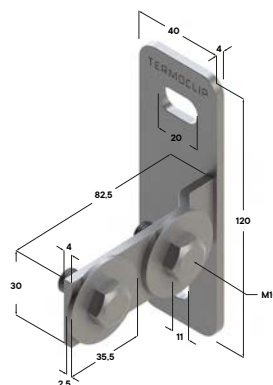
Фланец торцевой продольный TEF L 38-40 4F2 M10
