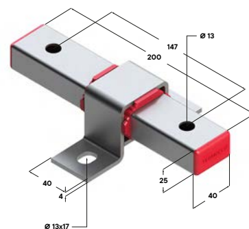
Опора скользящая TSA B40x25 F2
