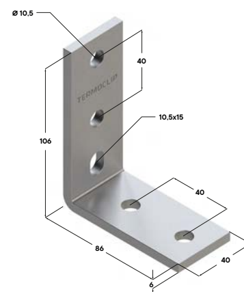
Уголок TA 90° 38-41 6F5
