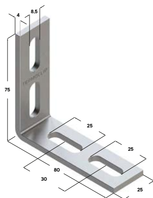
Уголок TA 90° 28 4F4
