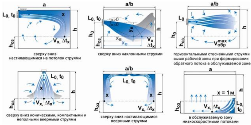
Рисунок Ж.1 - Основные схемы подачи приточного воздуха
