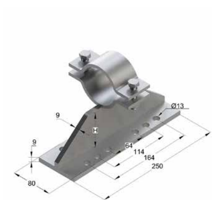
Опора трубная TPF 1-1 250x80 Н 85/140 9F 50x6F
