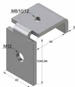
Угол седельный TAF 5F2
