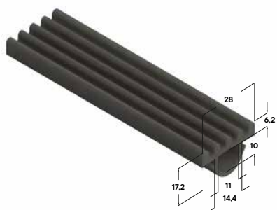
Вставка изолирующая TRI SC 28
