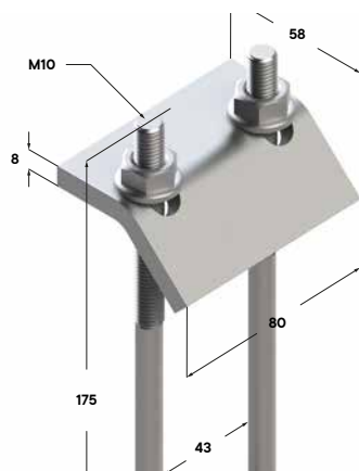
Зажим балочный 41 (124) M10
