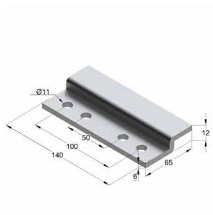
Скоба направляющей трубной опоры TBG 6F4
