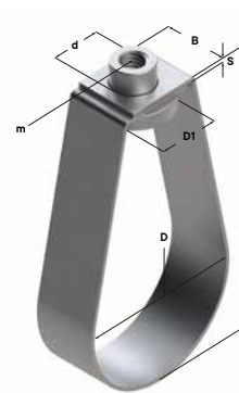
Хомут спринклерный с гайкой TS
