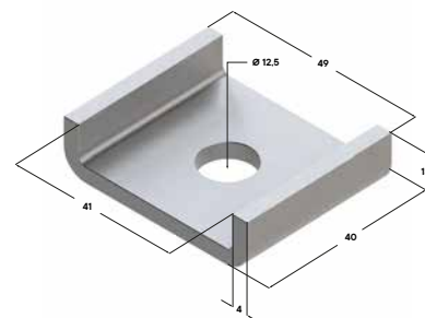
Шайба седельная TSW 38-41x40 4F
