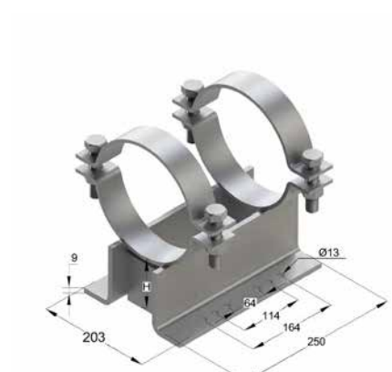
Опора трубная TPF 2-2
