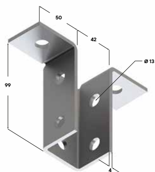
Соединитель 3D фланцевый TFC 38-41 4F8
