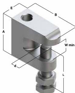
Струбцина F1
