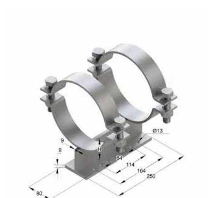
Опора трубная TPF 1-2 250x80 Н 85/106 140 9F 50x6F
